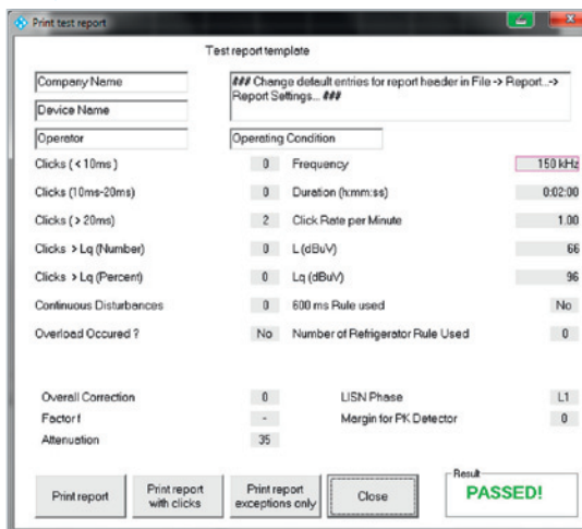
Измерение кратковременных помех — обработка данных/ отчет.
