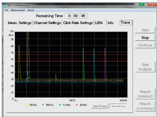
Анализ кратковременных помех — пример 1.
