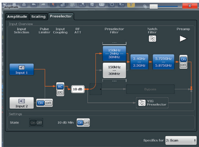
Возможность конфигурирования преселектора на входе приемника.
