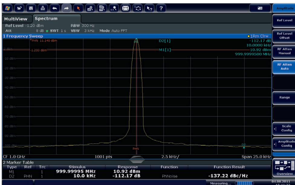
Фазовый шум -137 дБн (1 Гц) при отстройке на 10 кГц от несущей 1 ГГц.
