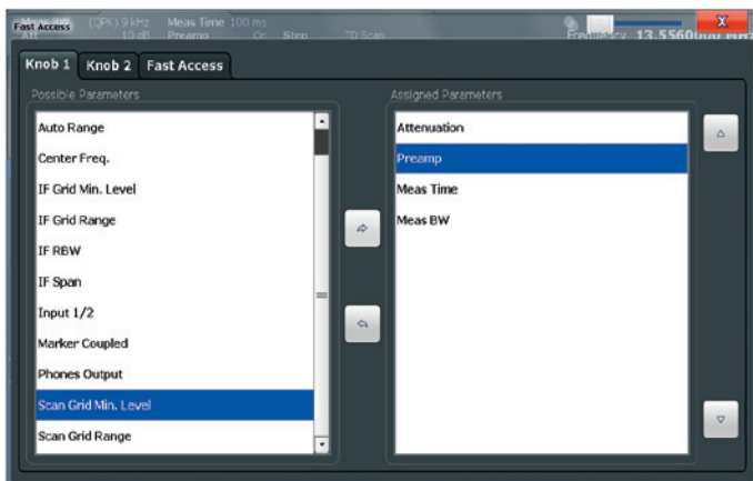
Выбор параметров для назначения функций для поворотных кнопок.
