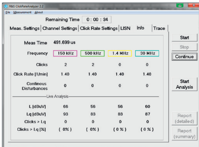
Анализ кратковременных помех — пример 2.
