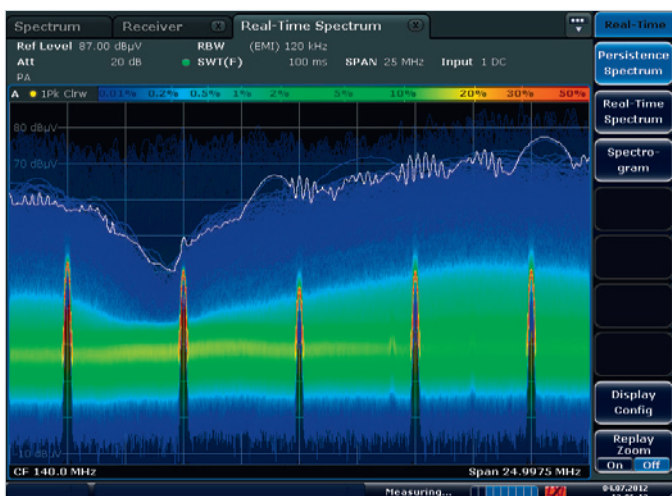
Спектр в режиме реального масштаба времени со скрытыми помехами
